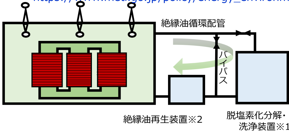
図 脱塩素化分解・洗浄技術を用いた循環洗浄法（※CDP洗浄法）の基本システム構成
